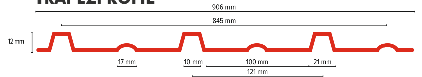
TRAPEZPROFIL
