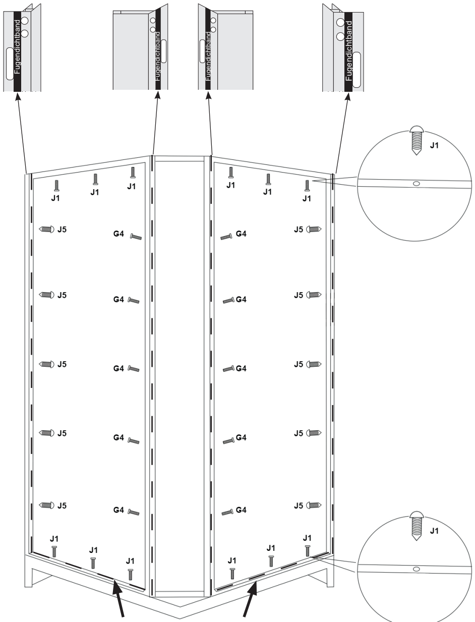
Fugendichtband zwischen Duschtasse und Rückwänden anbringen
