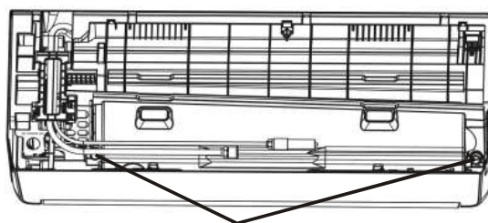
Odvodni otvori
