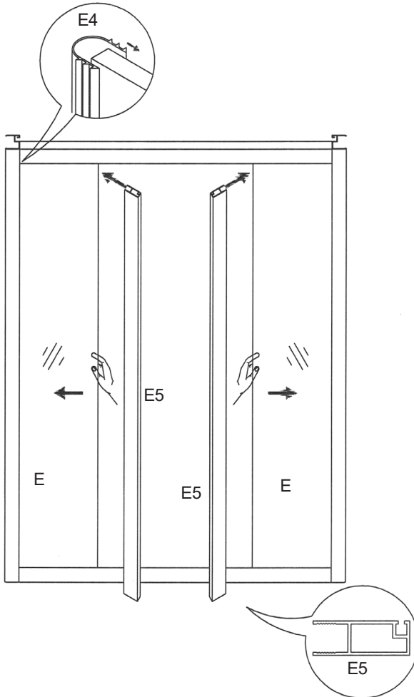
U-Dichtung Frontscheiben
