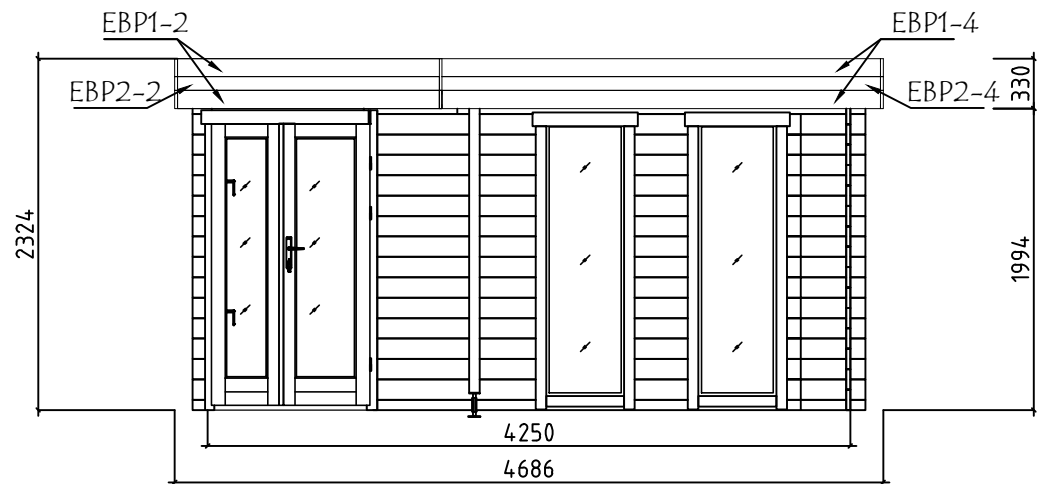
SEITENANSICHT (RECHTS) - SIDE VIEW (RIGHT)
