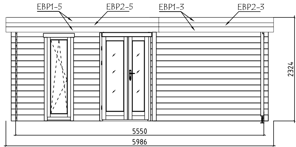
VORDERANSICHT-FRONT VIEW
