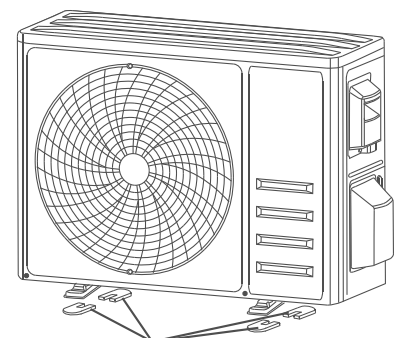
Coloque 4 placas de borracha (opcionais)
