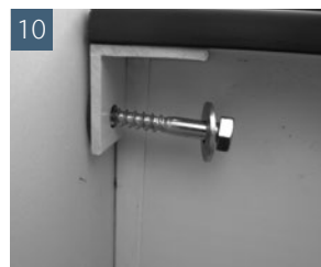
Schraube mit Beilagscheibe in Spiraldübel eindrehen
