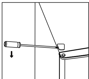
Schritt 3: Linke Abdeckung entfernen.
