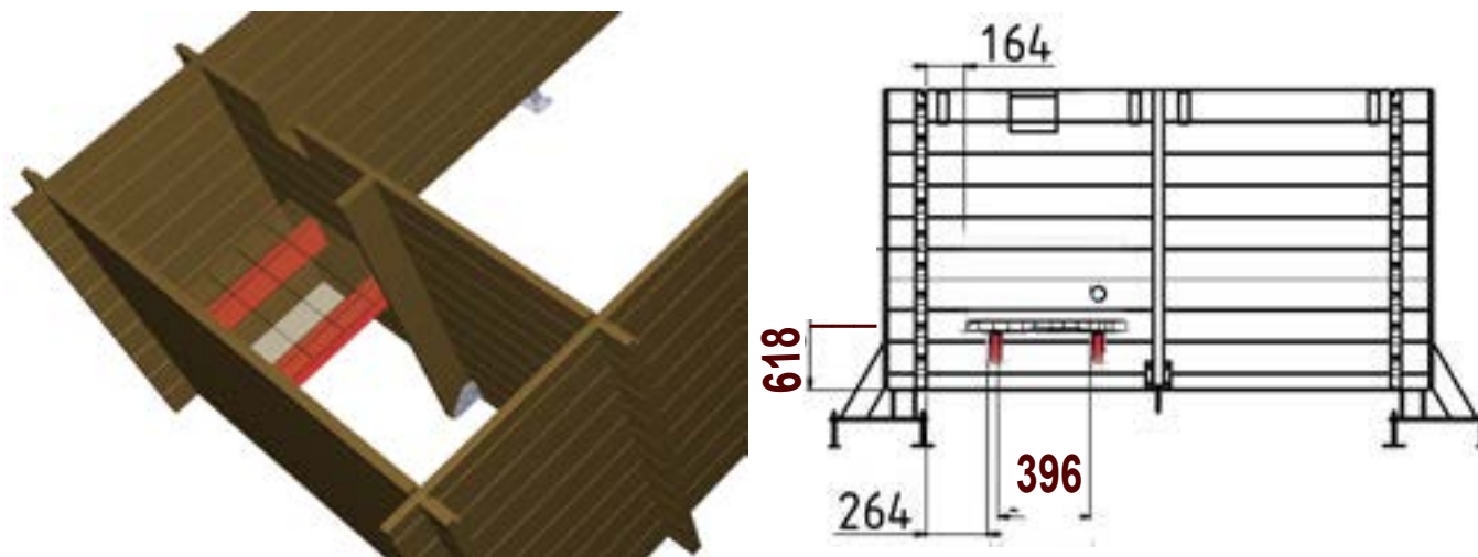
Abbildung 14 – Positionierung der Stützstreben des Box-Bodens
