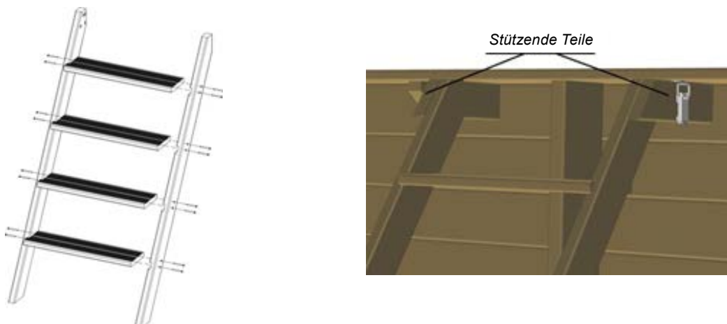
Abbildung 36 – Montage der Außentreppe aus Holz
