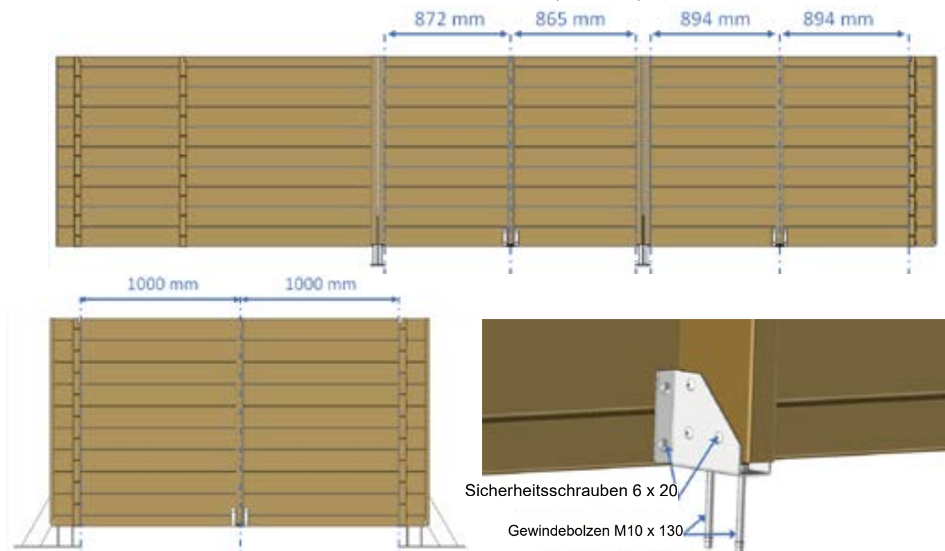
Abbildung 12 – Montage der Bodenanker für die Streben
