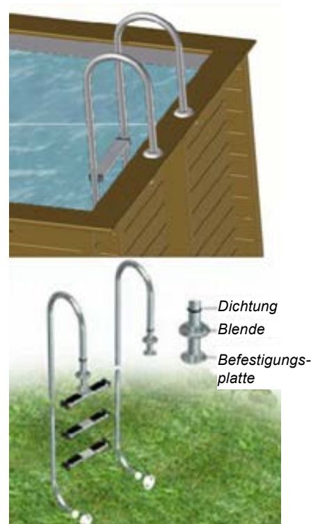
Abbildung 35 – Montage der Leiter
