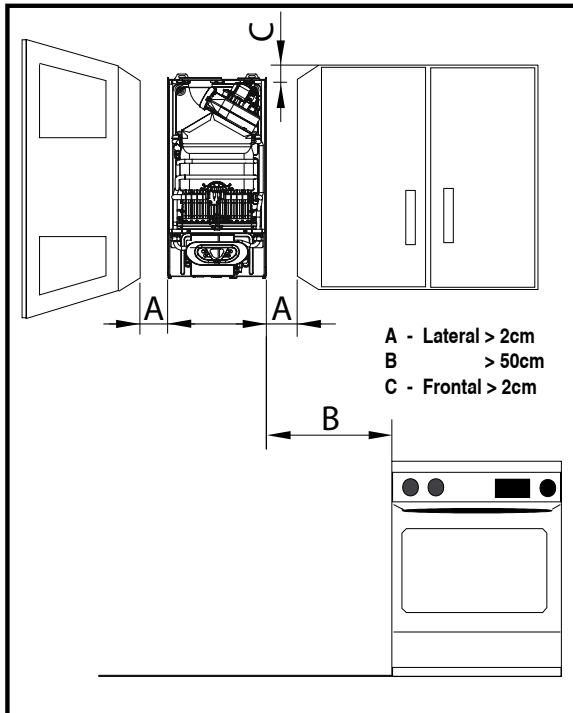
fig. 7 - Distancias mínimas
