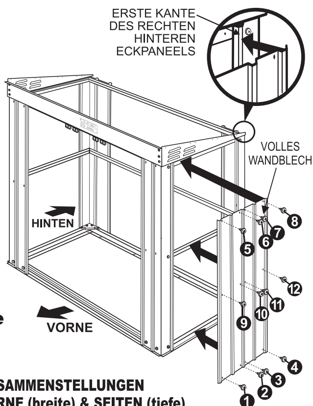
Diagramm 13A 3' tiefe Hütte
