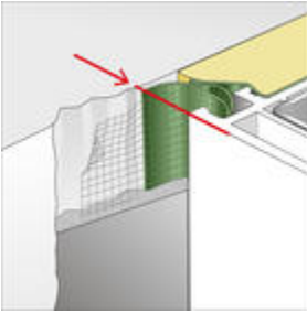
Bild 11: Einputzgitter in Mörtelbett eingelegt
