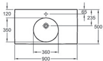
Preciosa II Waschtisch 900mm mit Hahnloch, ohne Überlauf Mod.- Nr. 12 32 92 01.10.2012/Th
