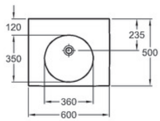
Preciosa II Waschtisch 600mm ohne Hahnloch, mit Überlauf Mod.- Nr. 12 32 61 01.10.2012/Th
