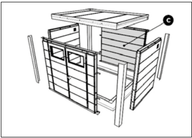
C Paroi / Wand / Wall / Wand
