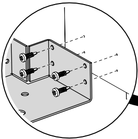
A + B Paroi / Wand / Wall / Wand
