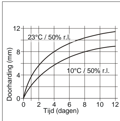
Schema 1: Uithardingsstijd voor Sikaflex®-295 UV
