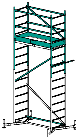
Grundgerüst + 1. Aufstockung Art.-Nr. 10091693 Art.-Nr. 10091703
