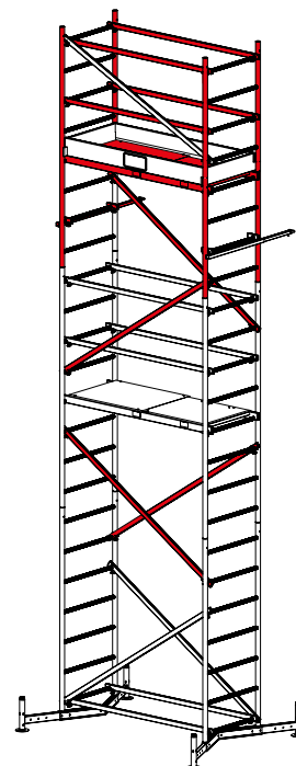
Grundgerüst + 1. Aufstockung + 2. Aufstockung Art.-Nr. 10091693 Art.-Nr. 10091703 Art.-Nr. 10091710
