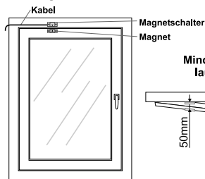
Frontansicht Fenster geschlossen
