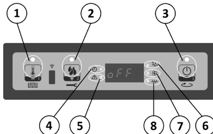
Fig. 3 - Pantalla: ledes encendidos
