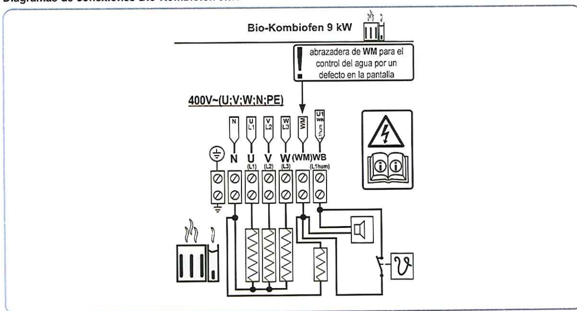
Diagramas de conexiones Bio-Kombiofen 9kW
