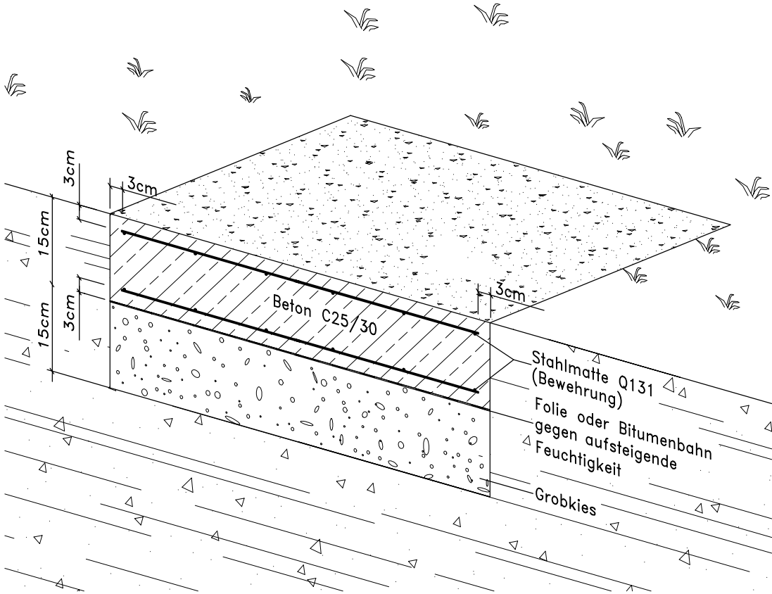
Schnitt A-A
