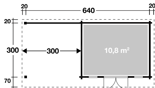
Trondheim 70-A XL mit Terrassenanbau 300 cm links
