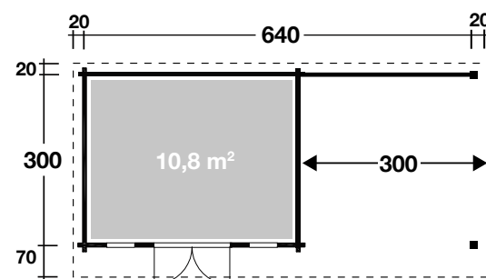
Trondheim 70-A XL mit Terrassenanbau 300 cm rechts
