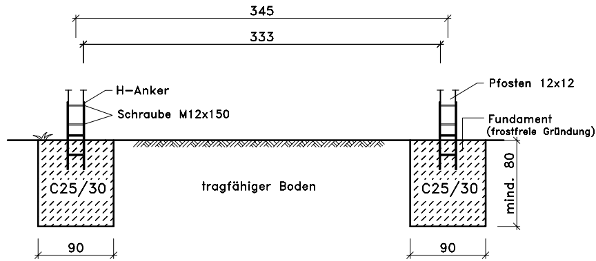
Schnitt A-A
