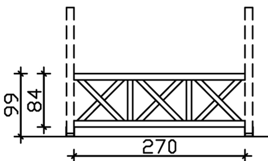
Bemassung
