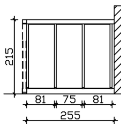
Bemassung
