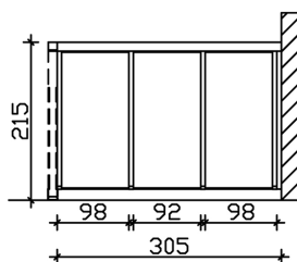
Bemassung
