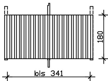
Bemassung
