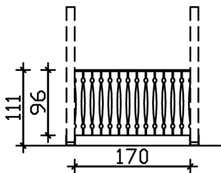
Bemassung
