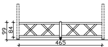
Bemassung
