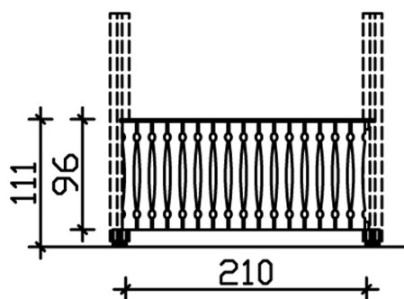
Bemassung
