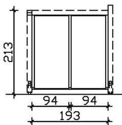
Bemassung
