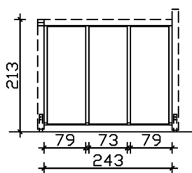
Bemassung
