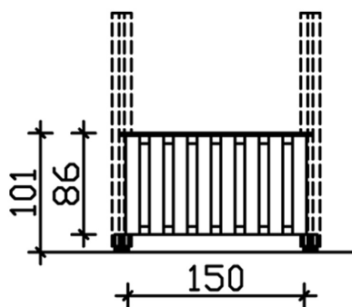
Bemassung
