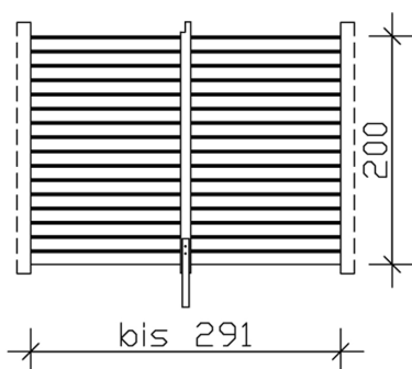
Bemassung
