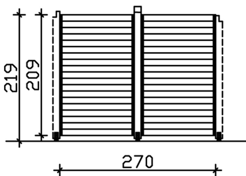
Bemassung
