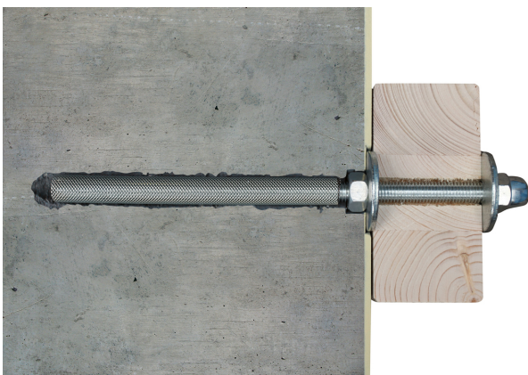
Querschnitt Wandbefestigung
