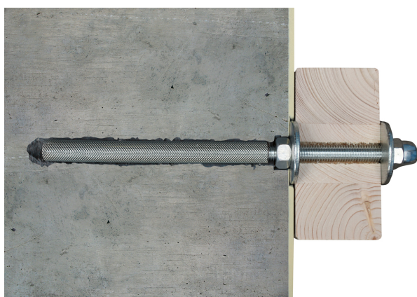
Querschnitt Wandbefestigung
