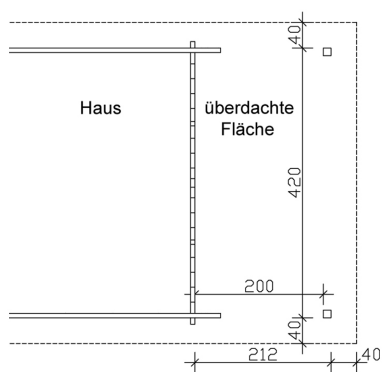
Grundriss
