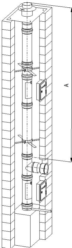
Bild 1: Aufbauhöhen
