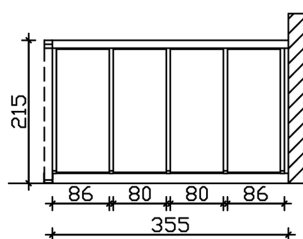
Bemassung
