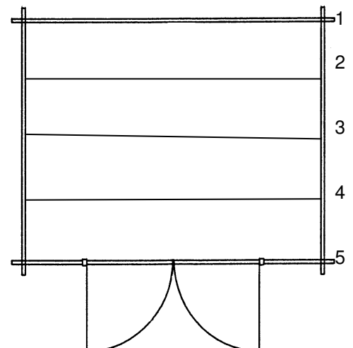
Grundriss und Fundamentplan (5 Fundamenthölzer)
