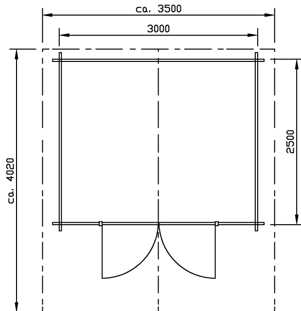
Grundriss und Fundamentplan (5 Fundamenthölzer)
