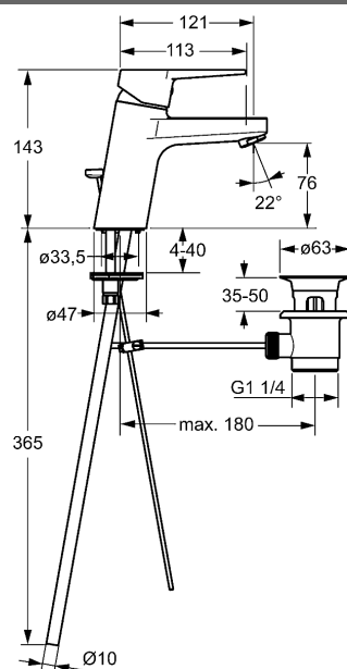
Produktzeichnung
