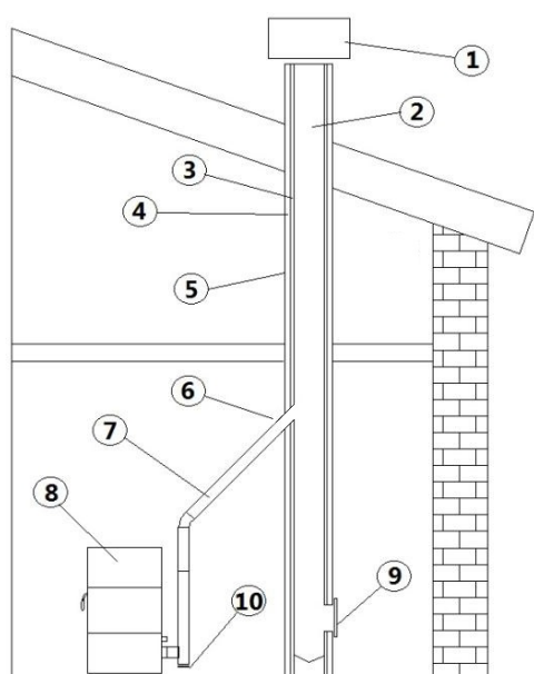
Fig. 5 - Bauteile Kamin
