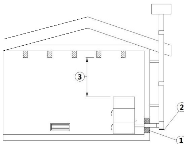
Fig. 13 - Beispiel 3
