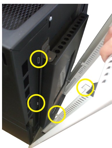
Fig. 21 - Montage Rahmen
