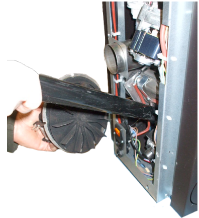
Fig. 78 - Phase 3
