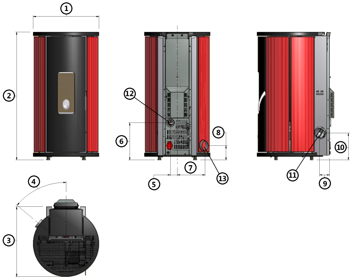
Fig. 17 - Allgemeine Abmessungen: Sfera 3 / Sfera 3 Plus / Globe
