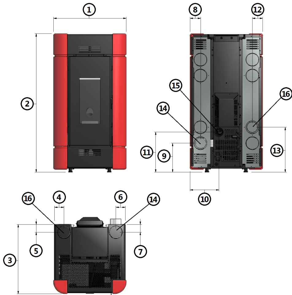
Fig. 15 - Allgemeine Abmessungen: Sire 3 Plus
