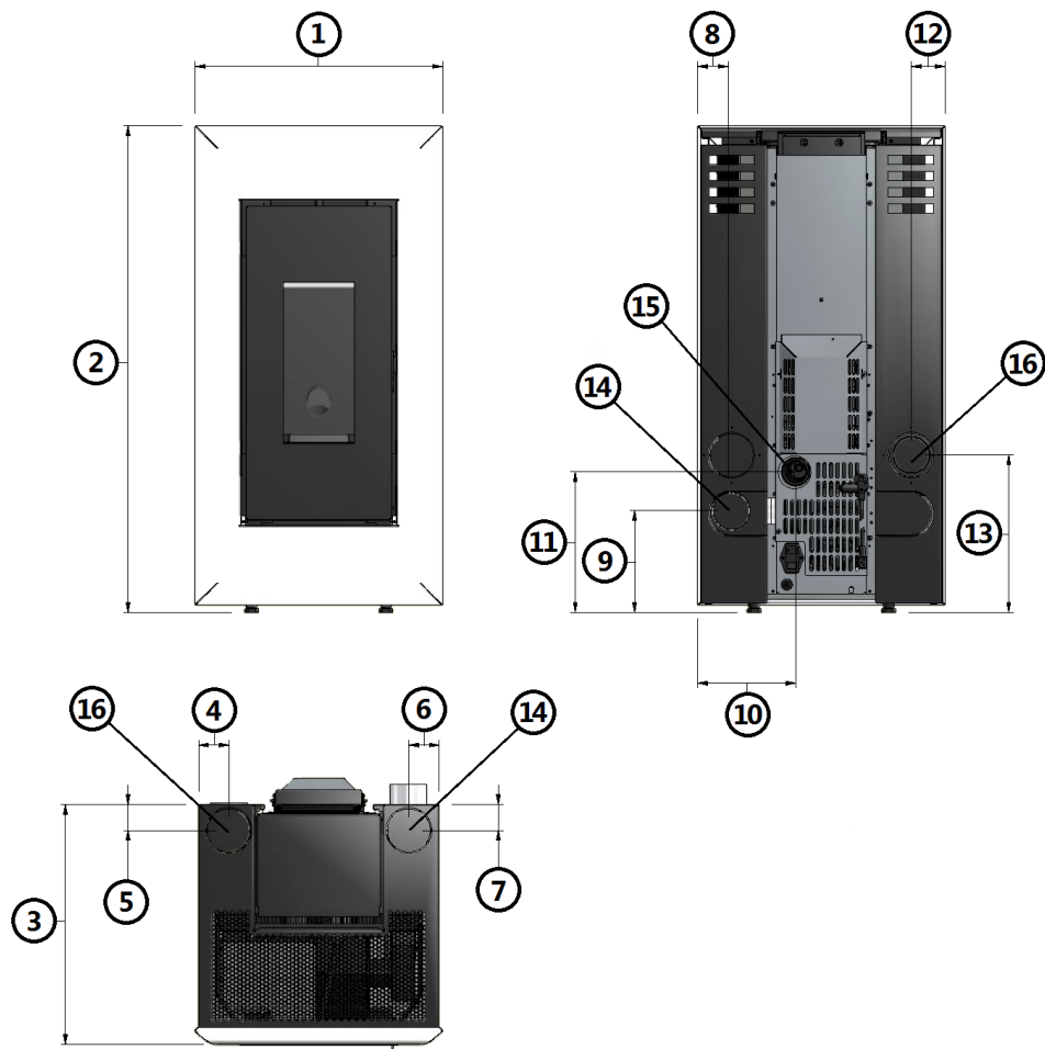
Fig. 14 - Allgemeine Abmessungen: Vega / Trend
