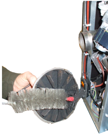
Fig. 77 - Phase 2
