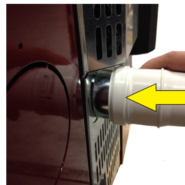
Fig. 10 - Phase 3
