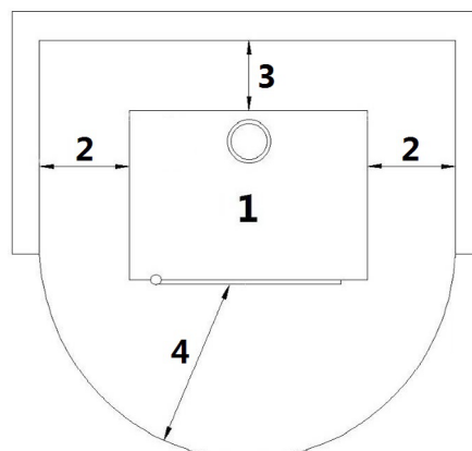
Fig. 20 - Allgemeine Installation
