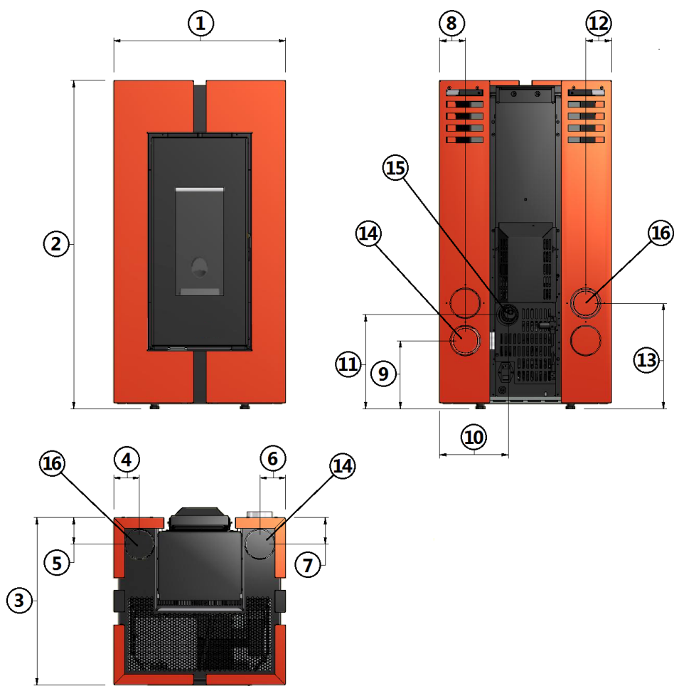
Fig. 16 - Allgemeine Abmessungen: Doge 3 Plus
