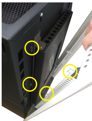
Fig. 35 - Montage Rahmen
