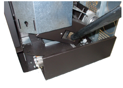
Fig. 73 - Reinigung Rauchgaskammer
