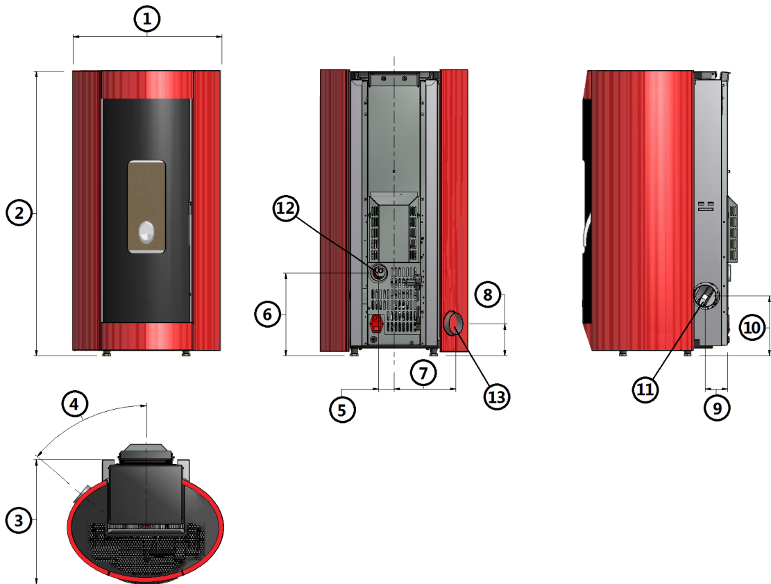
Fig. 19 - Allgemeine Abmessungen: Elise 3 Plus
