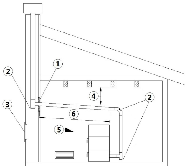
Fig. 12 - Beispiel 2
