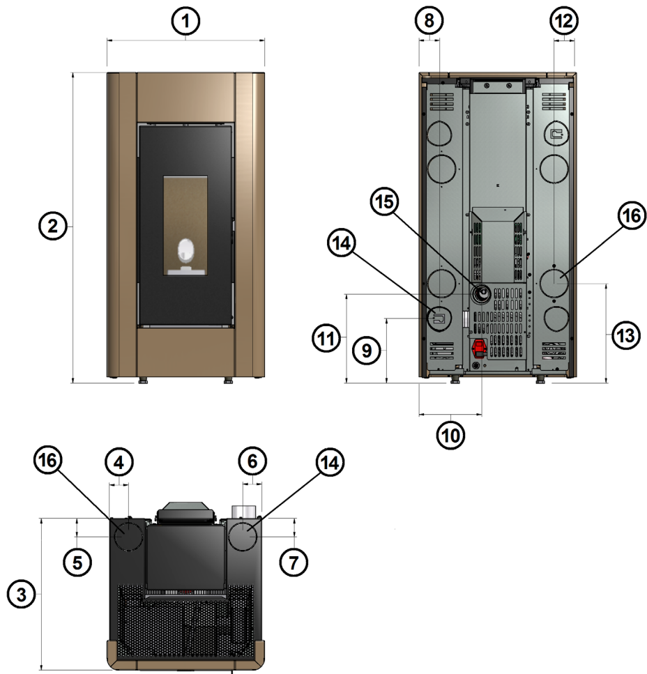
Fig. 18 - Allgemeine Abmessungen: Prince 3 / Prince 3 Plus
