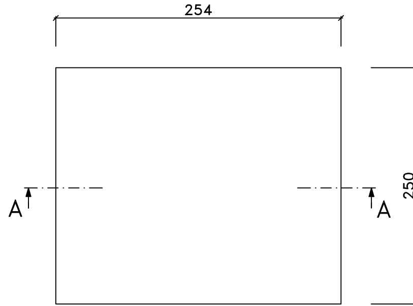
Frontseite
