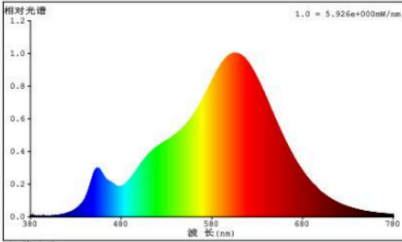
光谱分布
