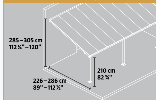
MARTINA – 3 Seitenwand
