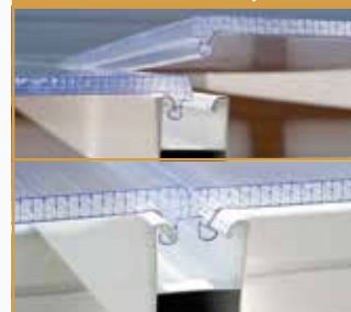
Klickverschluss Dachsystem
