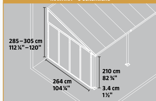
MARTINA – 3 Seitenwand
