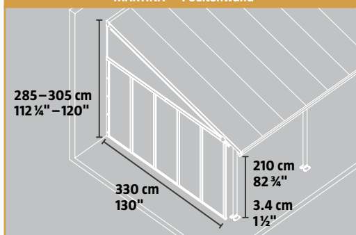
MARTINA – 4 Seitenwand
