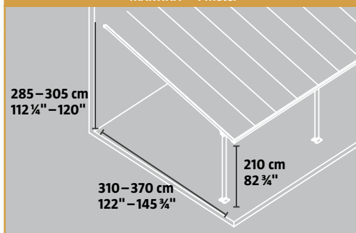
MARTINA – 4 Seitenwand
